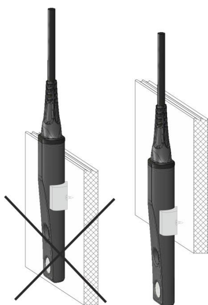
Fig. 1 Montage/Montage/Mountin/ Montaje
