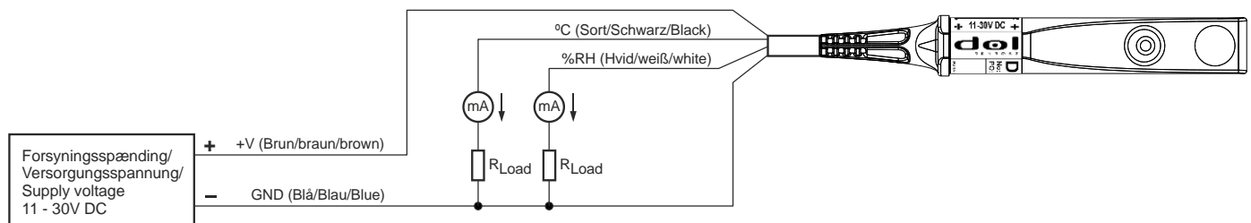
Fig. 3 Tilslutning/Anschluss/Connection/Conexión
